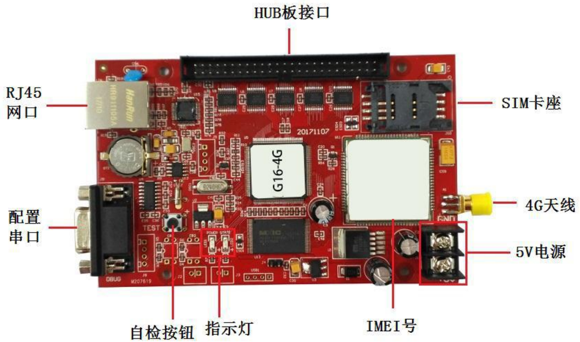
图 1-1 产品结构图
