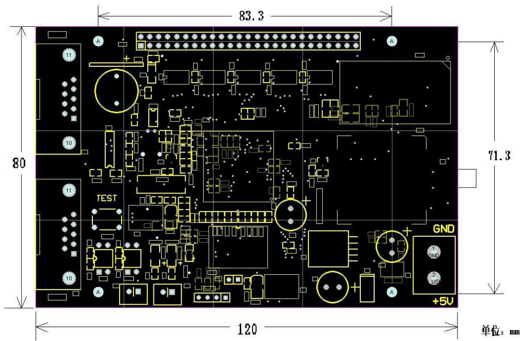
图 1-6 G16-4G 安装尺寸
