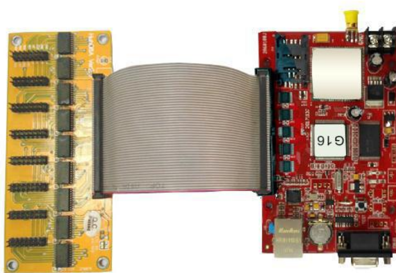
图 1-5 G16-4G 接 HUB 转接版示意图
