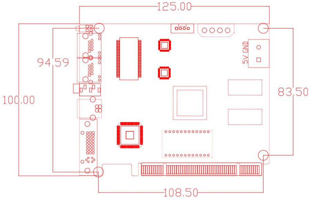
V9 孔位图
