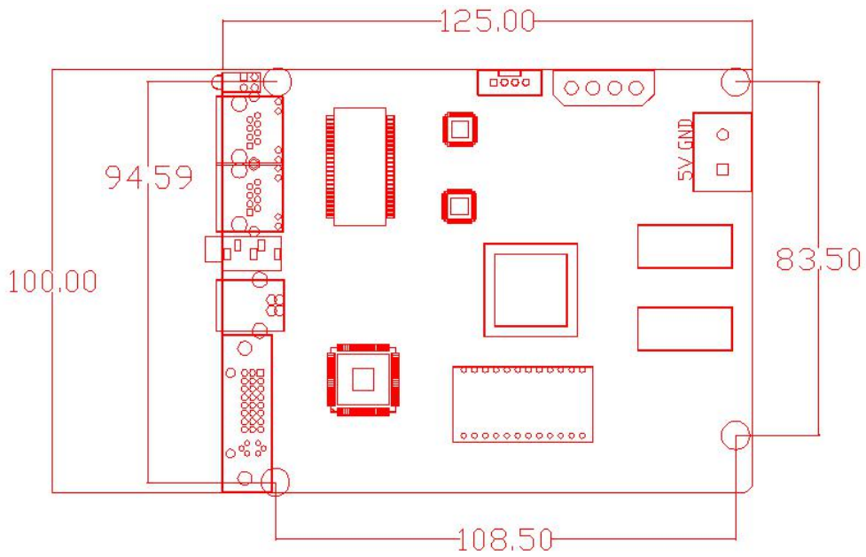
V9BOX 孔位图
